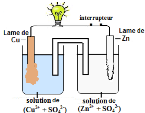
schéma (II): au cours du fonctionnement
