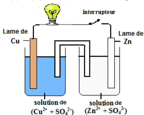
schéma (I): avant le fonctionnement
